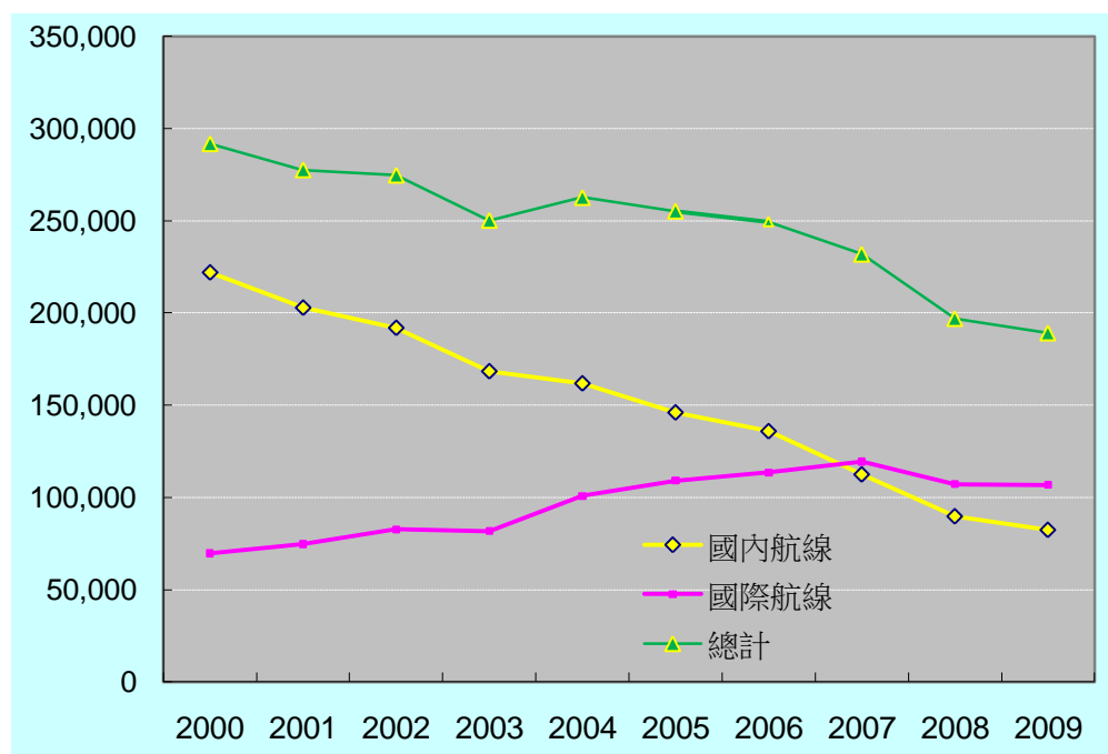
圖11： 2000-2009 年間我國民用航空運輸業飛行班次變化圖
