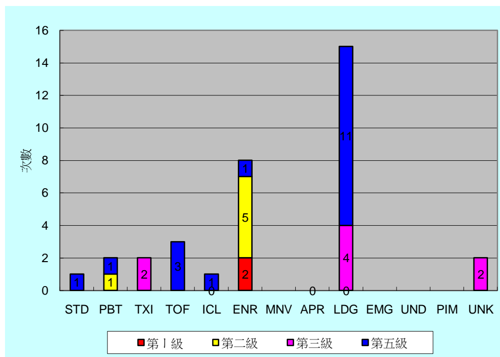
圖23： 2000-2009 國籍民用航空運輸業飛機飛航事故發生飛航階段次數（ICAO 飛航階段定義）
