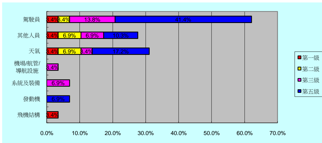
圖25： 2000-2009 國籍民用航空運輸業飛機各級飛航事故發生原因 (Causes/factors) 分類統計
