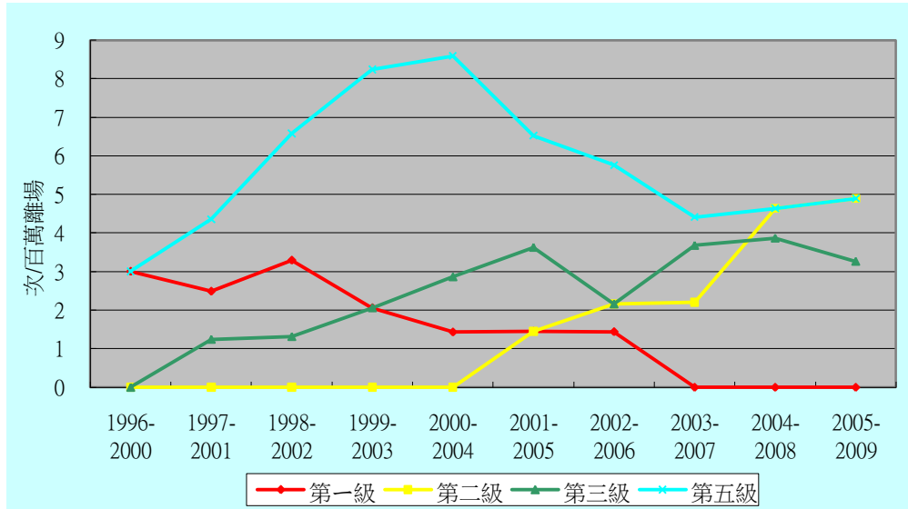
圖21： 國籍民用航空運輸業飛機飛航事故率（百萬離場）5年移動平均線（飛安會分類）
