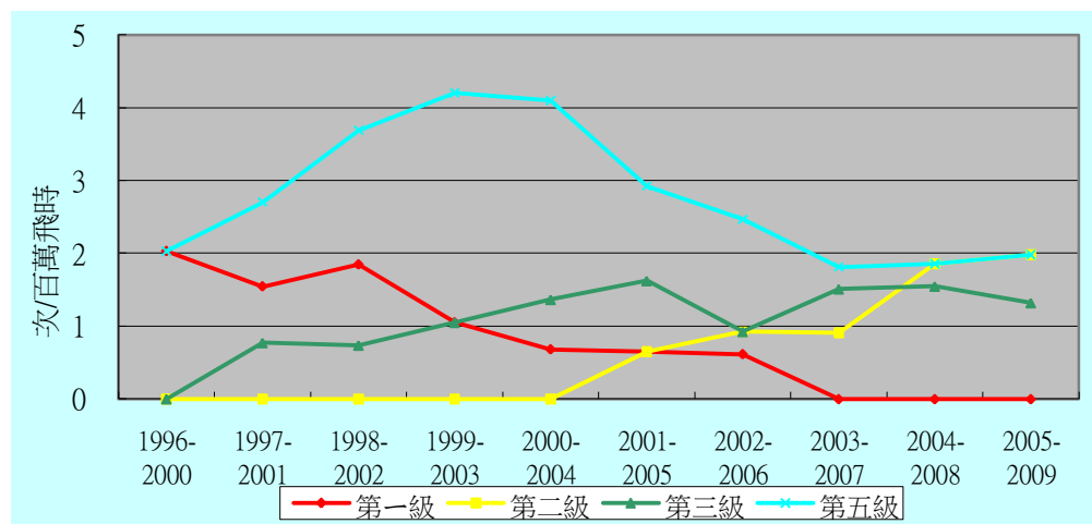
圖20： 國籍民用航空運輸業飛機飛航事故率（百萬飛時）5 年移動平均線（飛
