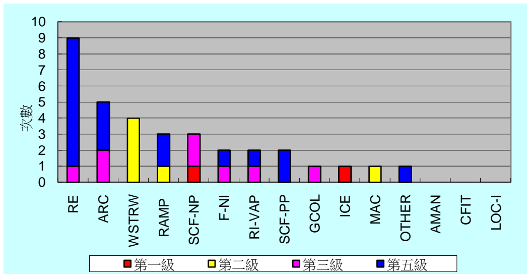
圖24： 2000-2009 國籍民用航空運輸業飛機飛航事故分類統計
