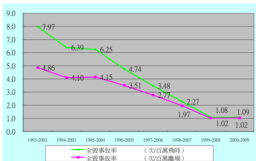
圖 17： 國籍民用航空運輸業渦輪螺旋槳飛機航空器全毀十年平均事故率
