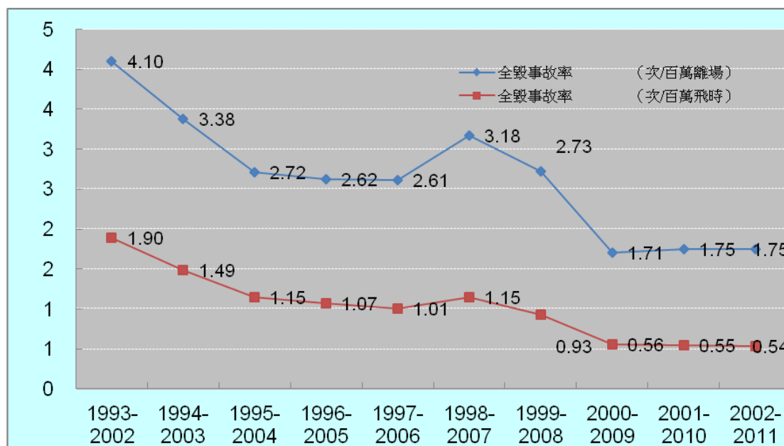
圖16： 國籍民用航空運輸業渦輪噴射飛機航空器全毀十年平均事故率
