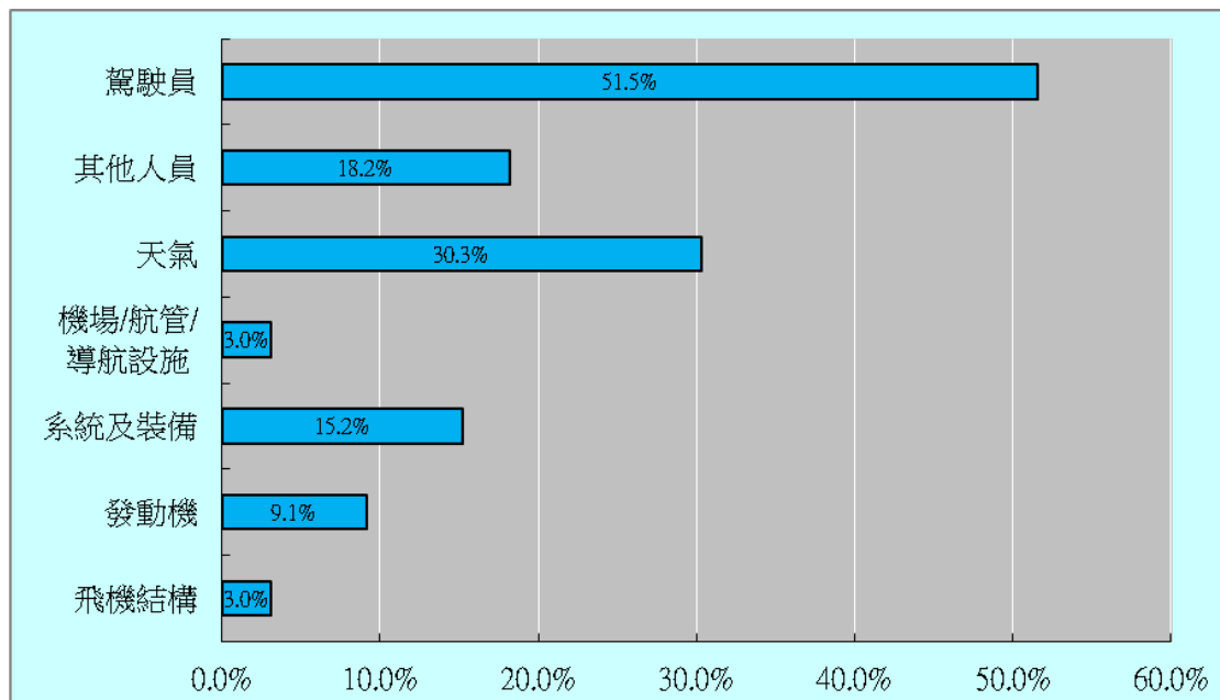
圖22： 2002-2011 年國籍民用航空運輸業飛機飛航事故發生原因分類統計
