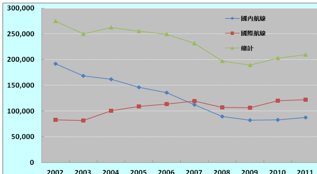
圖11： 2002-2011 年間我國民用航空運輸業飛行班次變化圖
