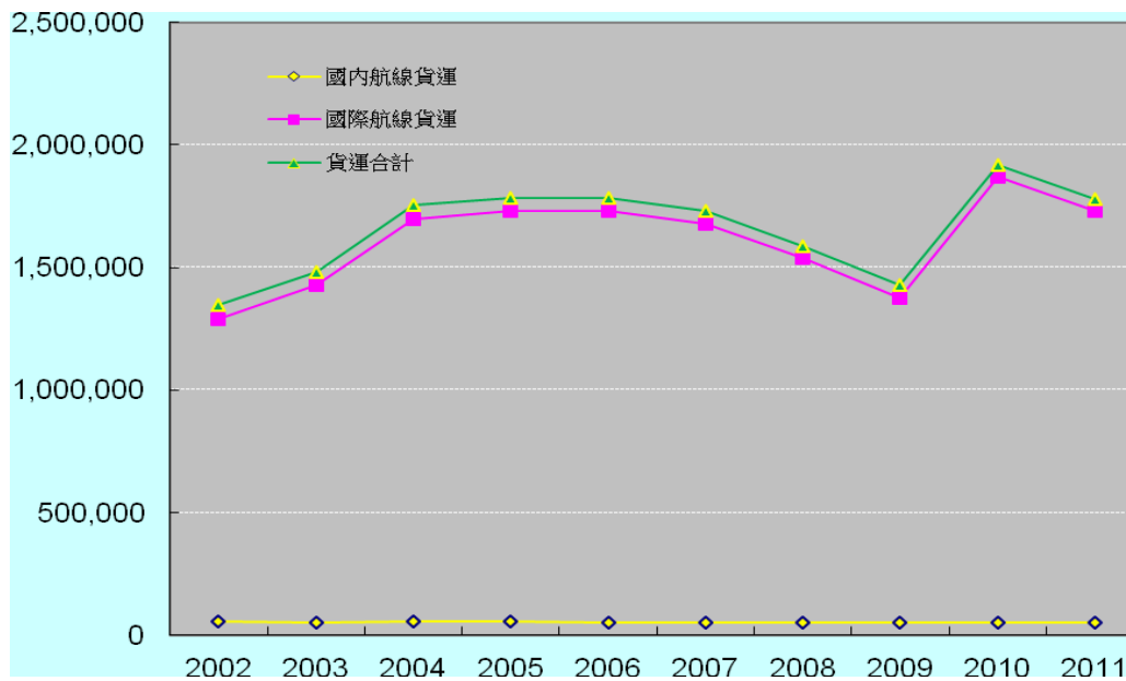
圖10： 2002-2011 年間我國民用航空運輸業貨運噸數變化圖
