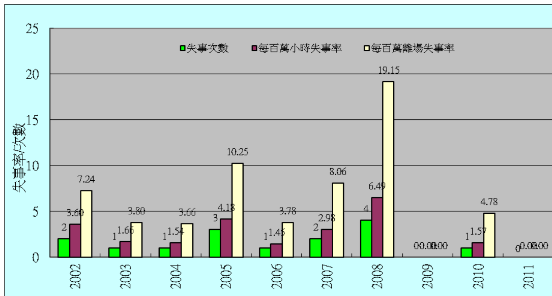
圖18： 2002-2011 年國籍民用航空運輸業失事次數及失事率
