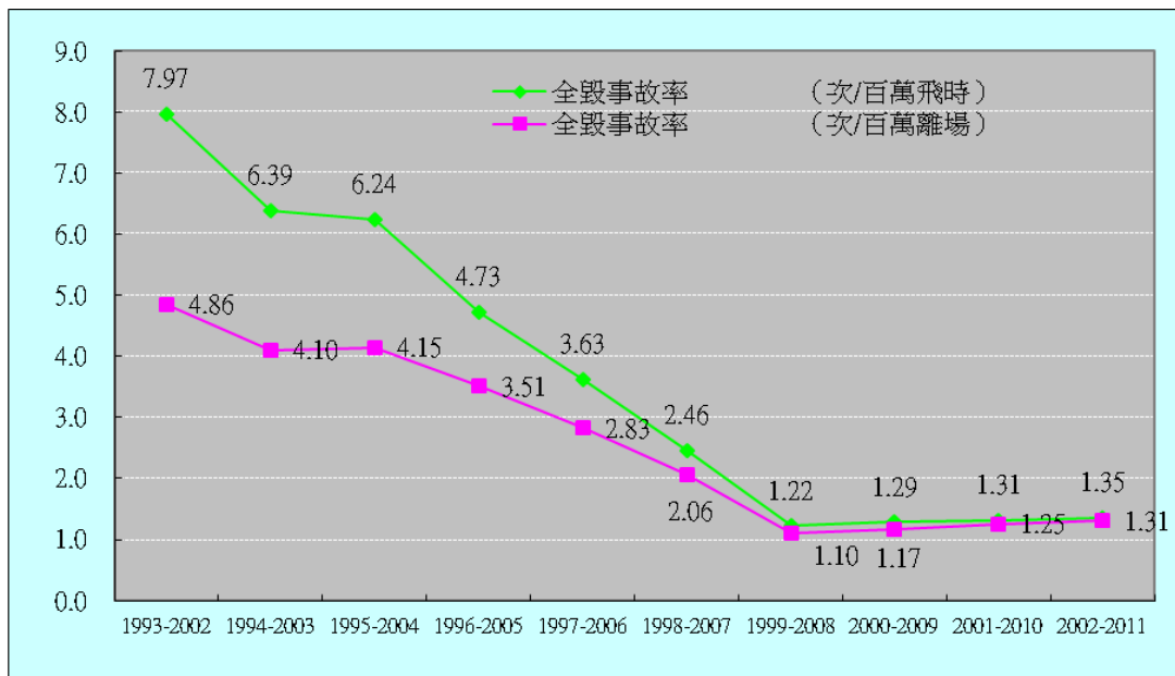
圖17： 國籍民用航空運輸業渦輪螺旋槳飛機航空器全毀十年平均事故率
