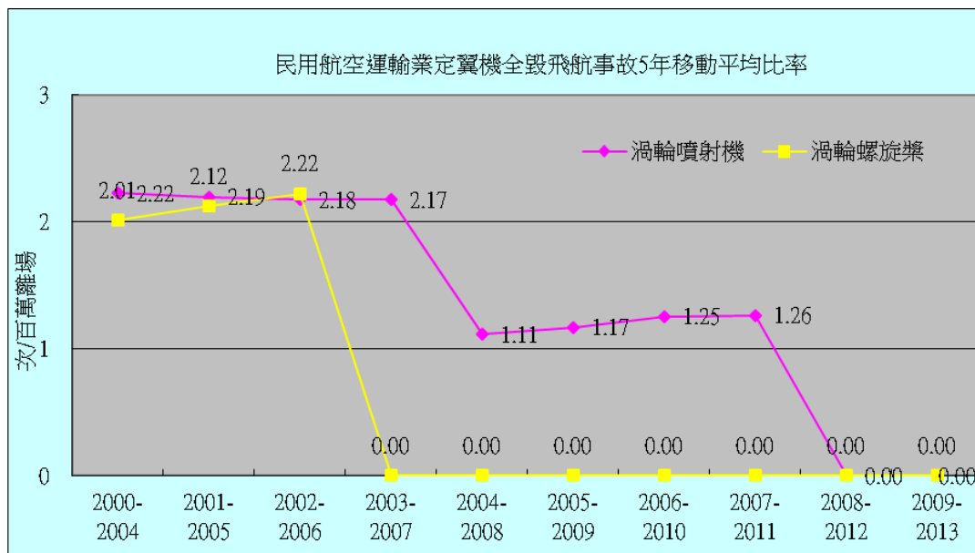
圖15： 國籍民用航空運輸業飛機全毀飛航事故率 5 年移動平均線
