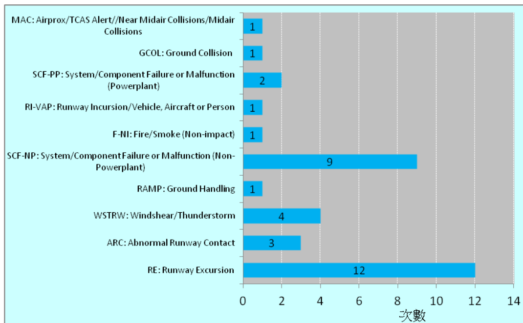
圖21： 2004-2013 年國籍民用航空運輸業飛航事故分類統計
