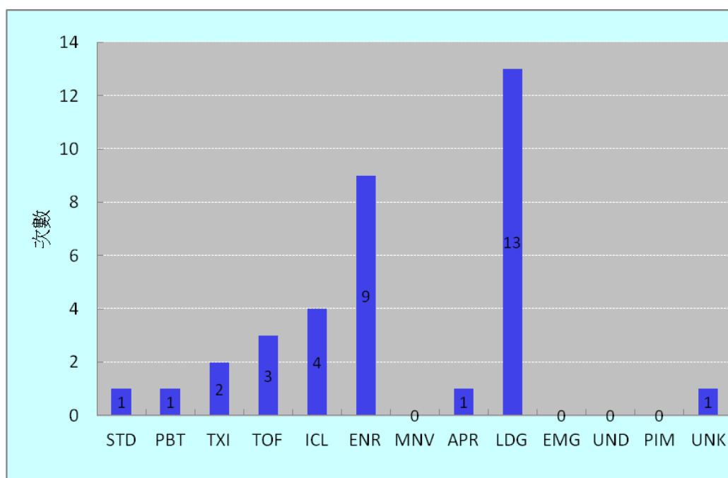
圖20： 2004-2013 年國籍民用航空運輸業飛航事故發生飛航階段次數
