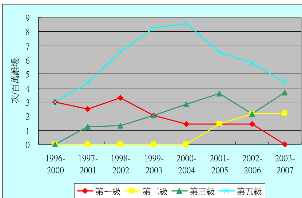
圖21： 國籍民用航空運輸業飛機飛航事故率（百萬離場）5年移動平均線（飛安會分類）
