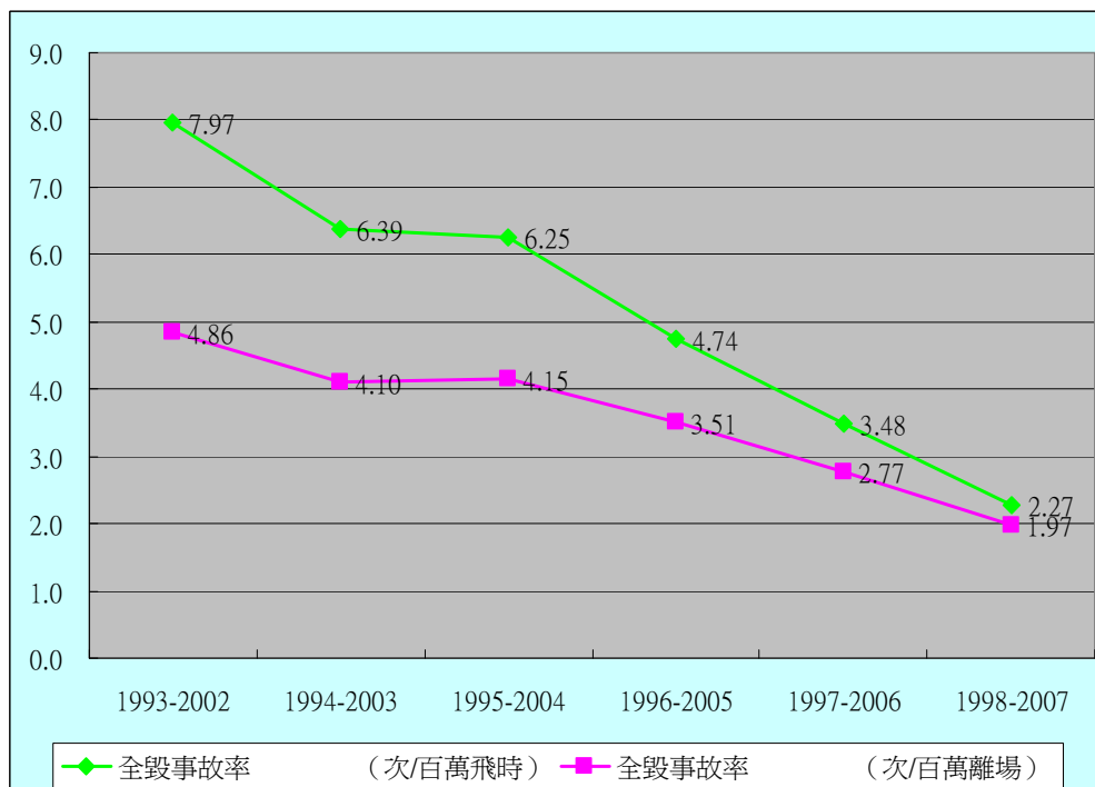
圖 17： 國籍民用航空運輸業渦輪螺旋槳飛機航空器全毀十年平均事故率
