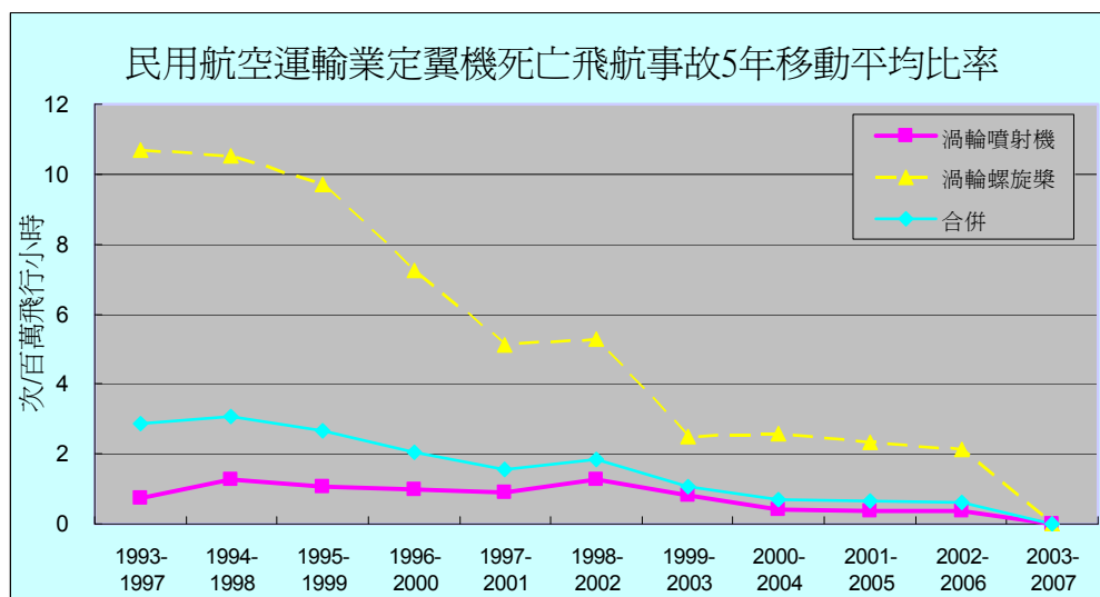
圖14： 國籍民用航空運輸業飛機致命飛航事故率 5 年移動平均線
