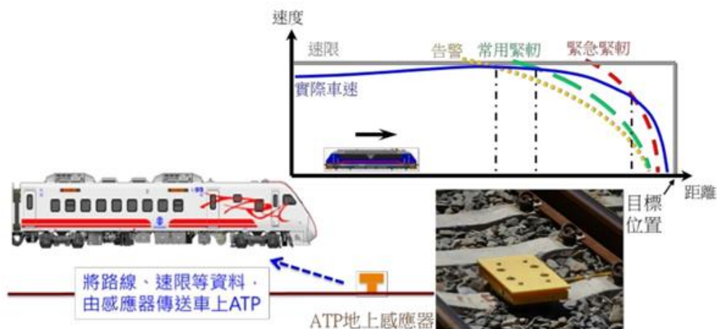
圖 1.9-1 ATP 系統運作原理與煞車曲線範例
