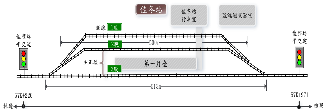
圖 1.12-1 佳冬站軌道線形
