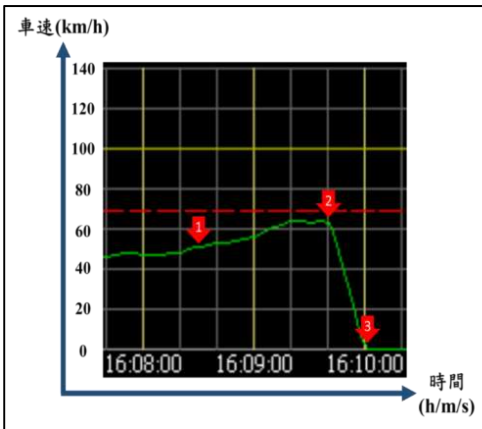
圖 1.12-1 事故列車 ATP 表
