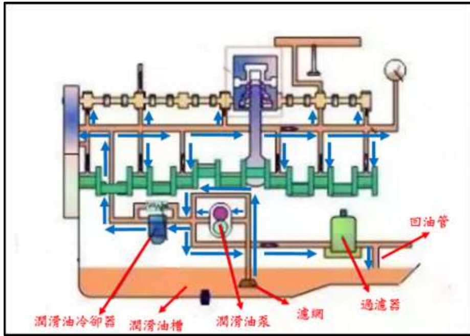
圖 1.7-5 潤滑油系統構造示意圖
