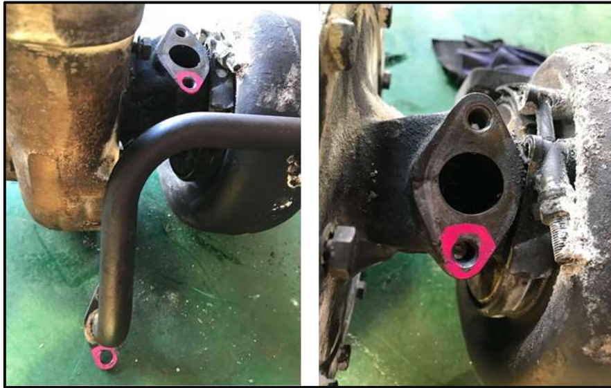
圖 1.7-11 回油管與渦輪增壓機接合處螺絲缺少（紅色標示）
