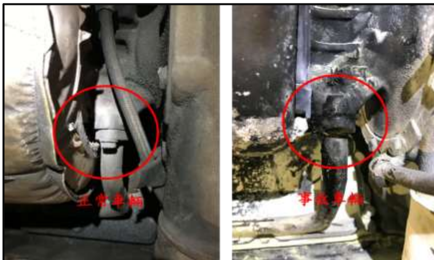
圖 1.7-8 回油管與渦輪增壓機接合情況比對
