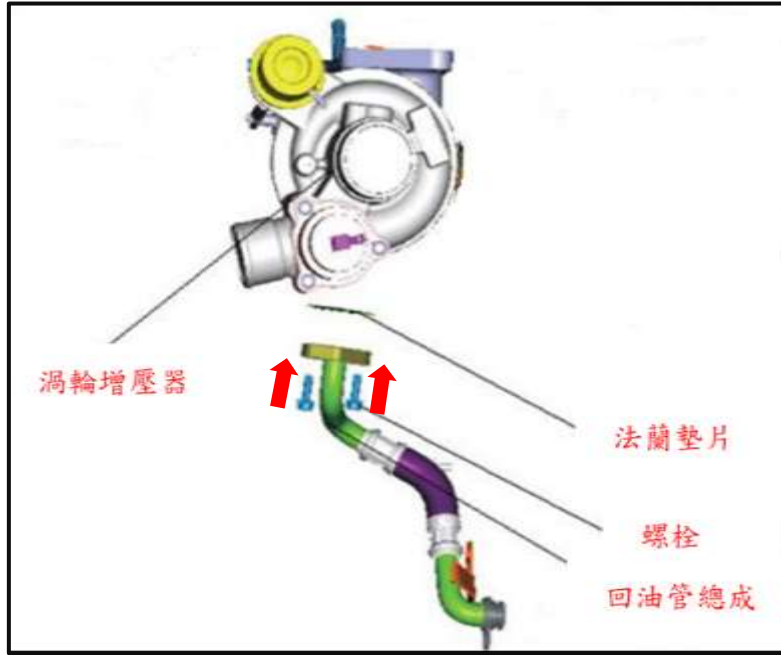
圖 1.7-7 潤滑油回油管與渦輪增壓機接合示意
