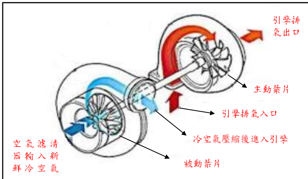
圖 1.7-4 渦輪增壓機運作示意圖
