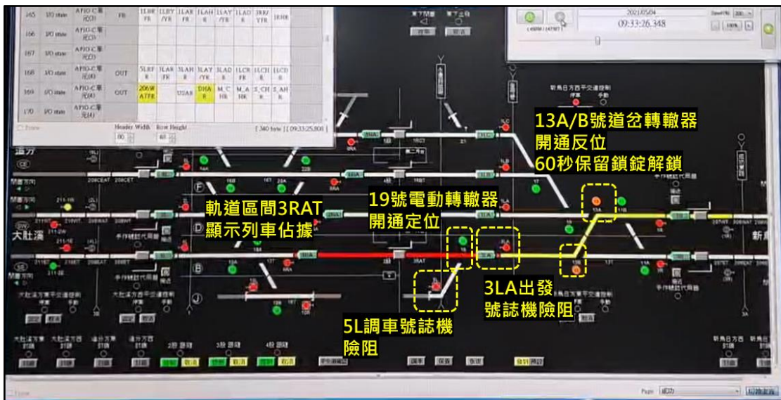
圖 1.9-10 0931:39 時成功站號誌運轉紀錄器狀態
