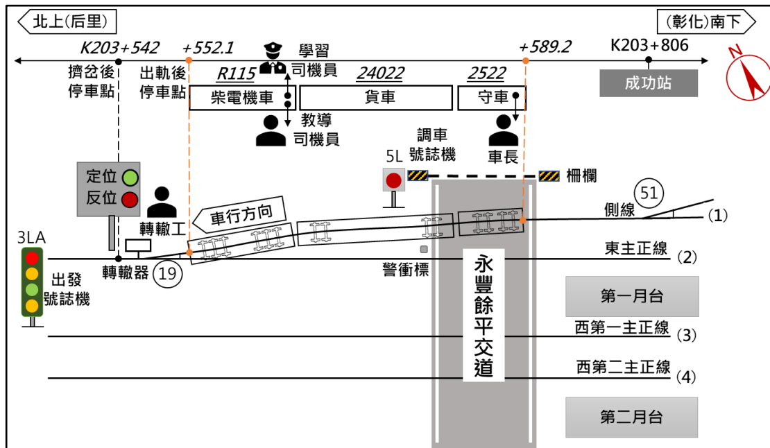
圖 1.1-3 第 7142 次車於成功站出軌後停車處
