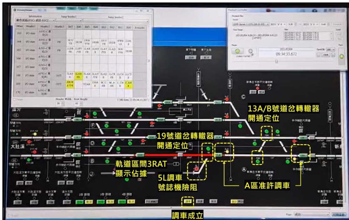
圖 1.9-13 0933:05 時成功站號誌運轉紀錄器狀態
