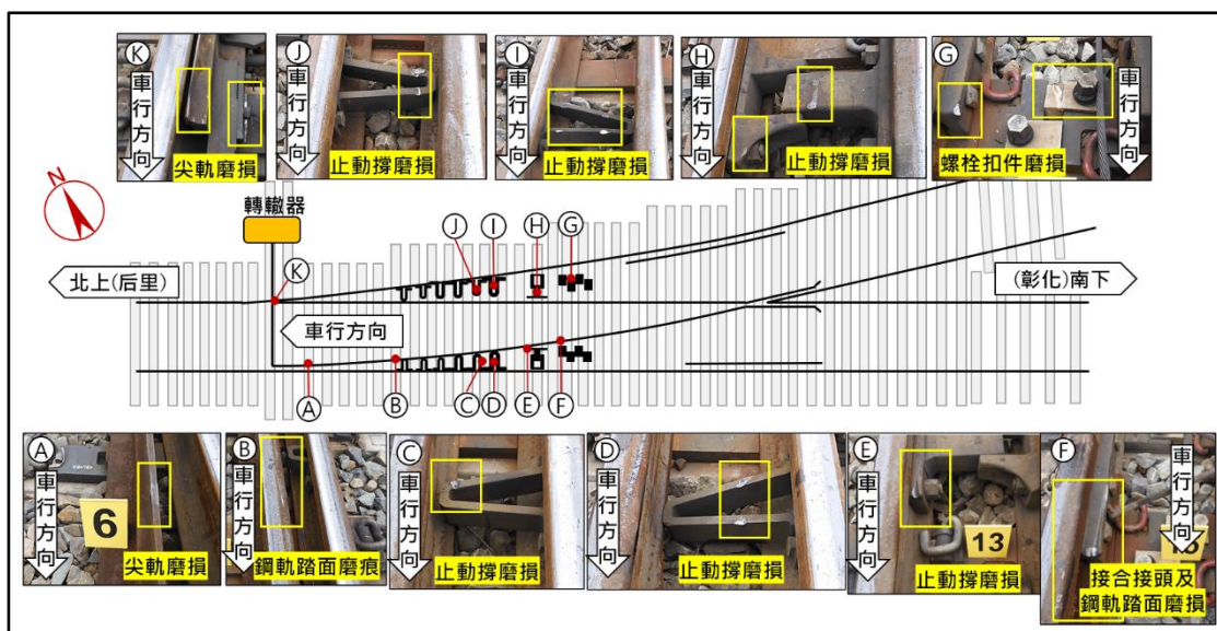
圖 1.4-1 19 號道岔損害情形 (1)
