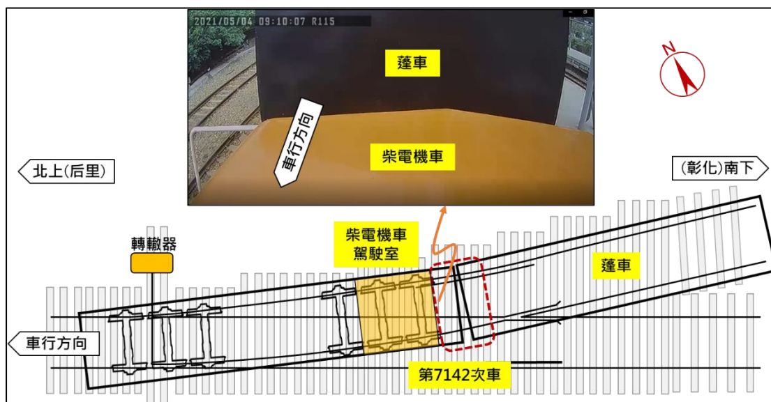
圖 1.13-1 第 7142 次車駕駛室行車影像紀錄器畫面
