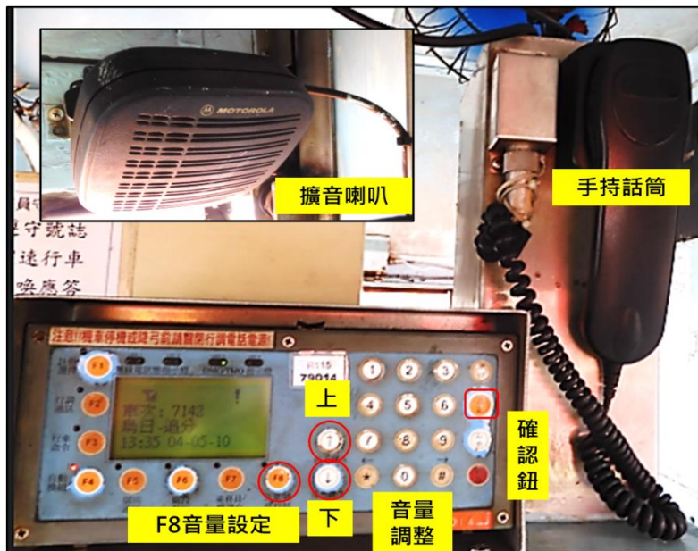
圖 1.11-1 行調無線電車上台及擴音喇叭
