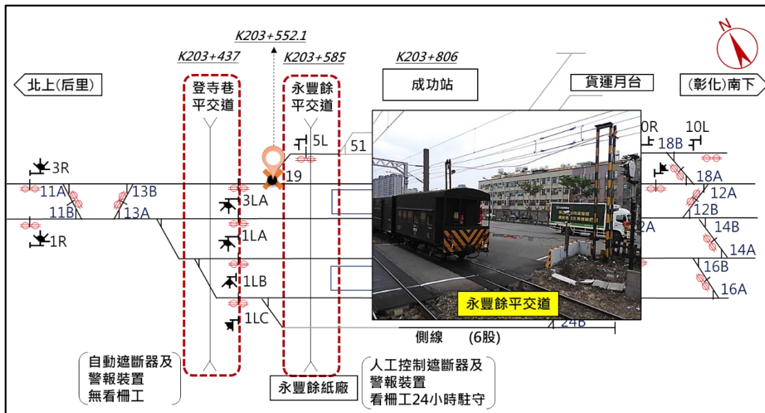
圖 1.10-1 成功站平交道配置示意圖
