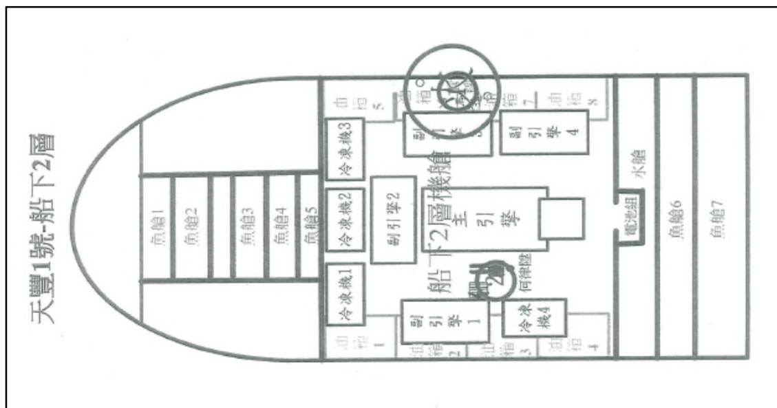
圖2 豐船起火點示意圖
