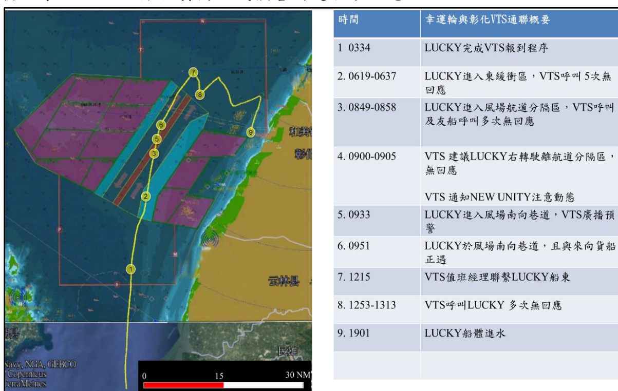
圖 4 彰化 VTS 與幸運輪通信時之相對位置圖
