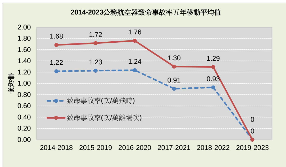
圖19 公務航空器致命事故率
