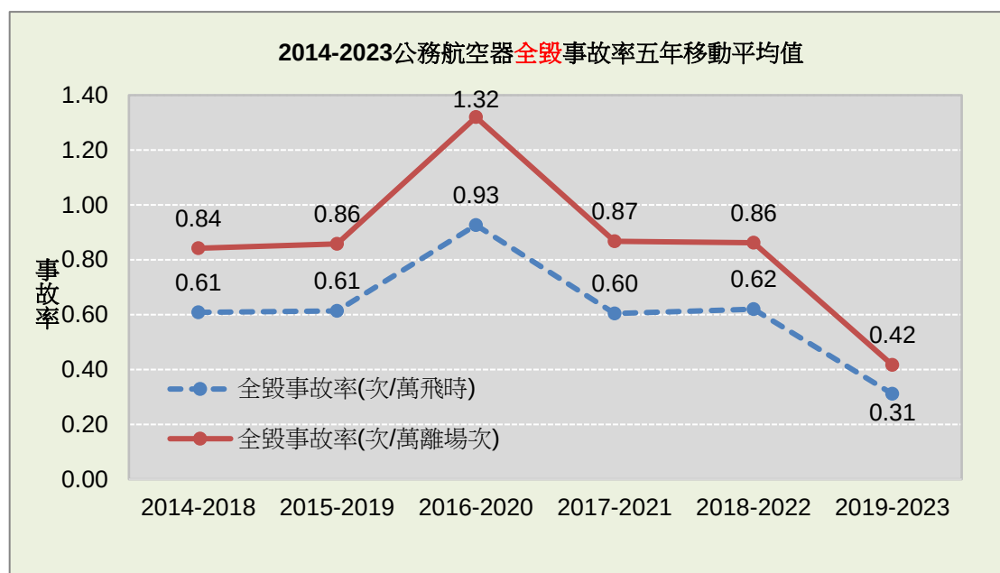
圖18 公務航空器全毀事故率
