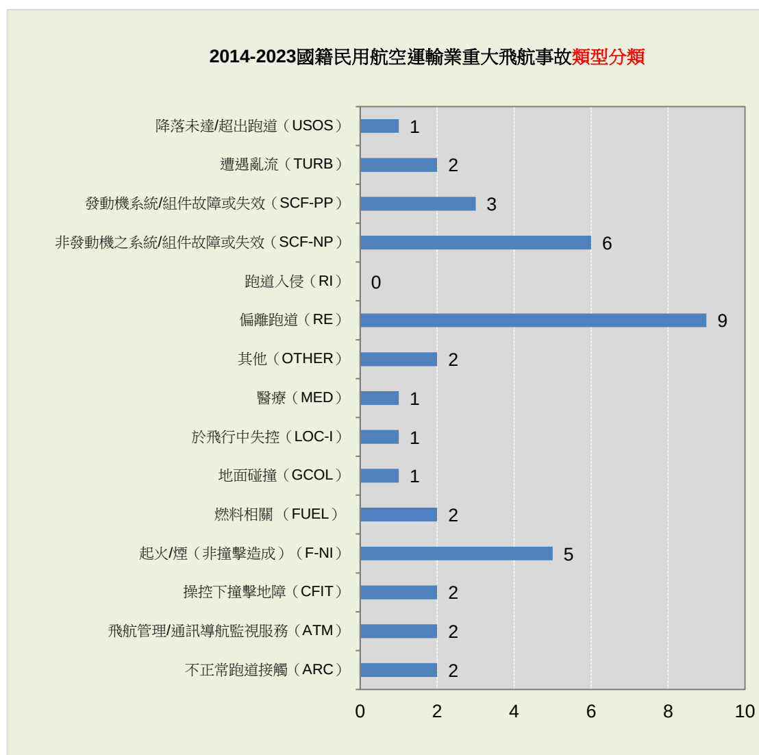
圖14 民用航空運輸業重大飛航事故類型分類統計
