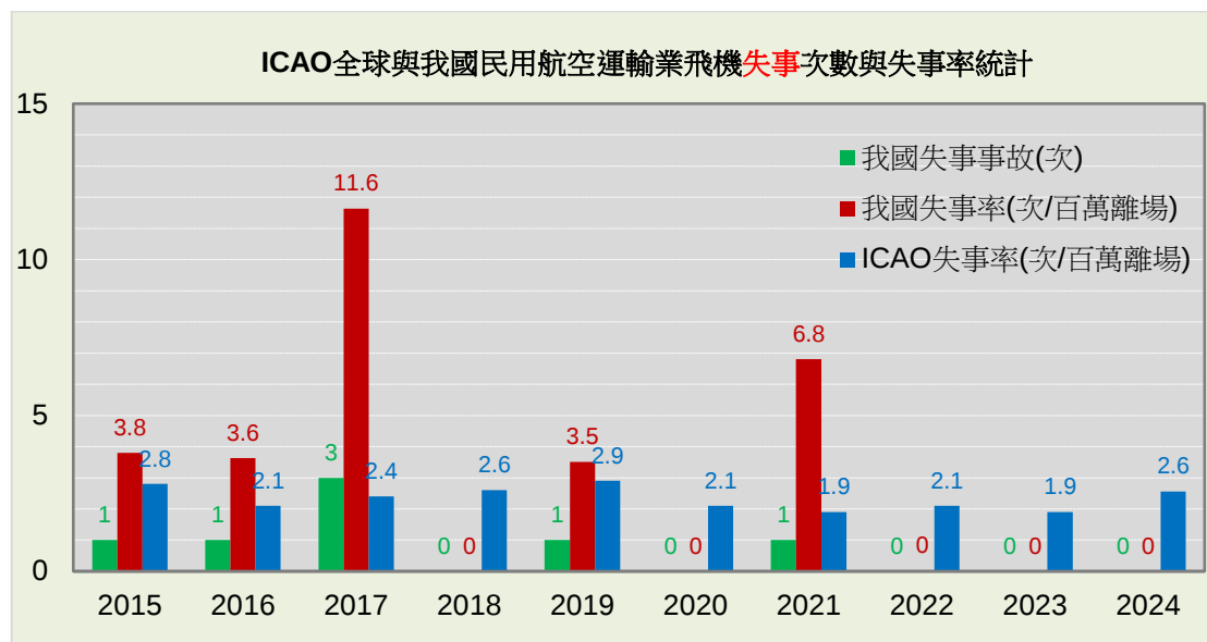
圖12 ICAO 與我國民用航空運輸業飛機失事統計
