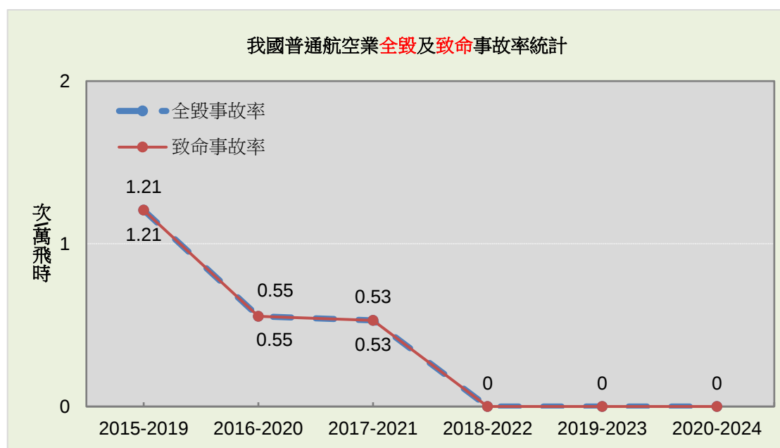
圖16 普通航空業航空器全毀及致命事故率
