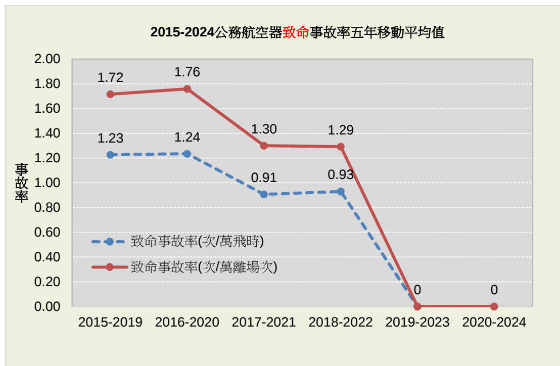
圖19 公務航空器致命事故率
