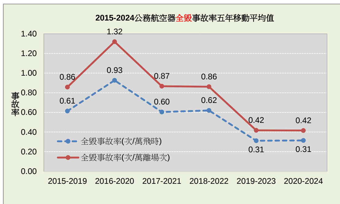
圖18 公務航空器全毀事故率
