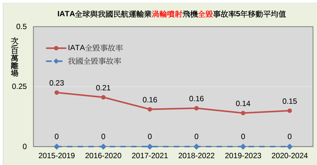
圖8 IATA 與我國民用航空運輸業渦輪噴射飛機全毀事故率
