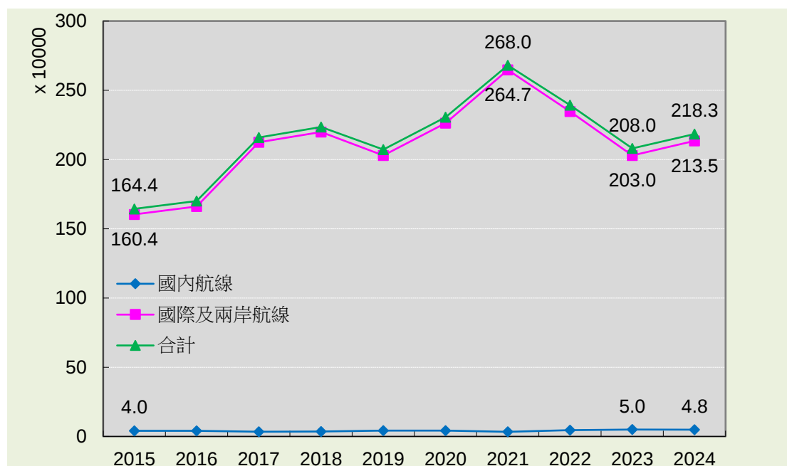
圖4 民用航空運輸業貨運量
