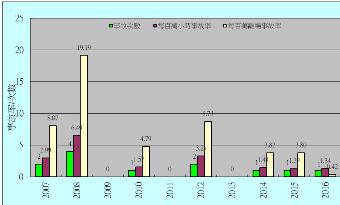
圖12： 2007-2016 年國籍民用航空運輸業 ICAO 定義 Accident 事故次數及事故率
