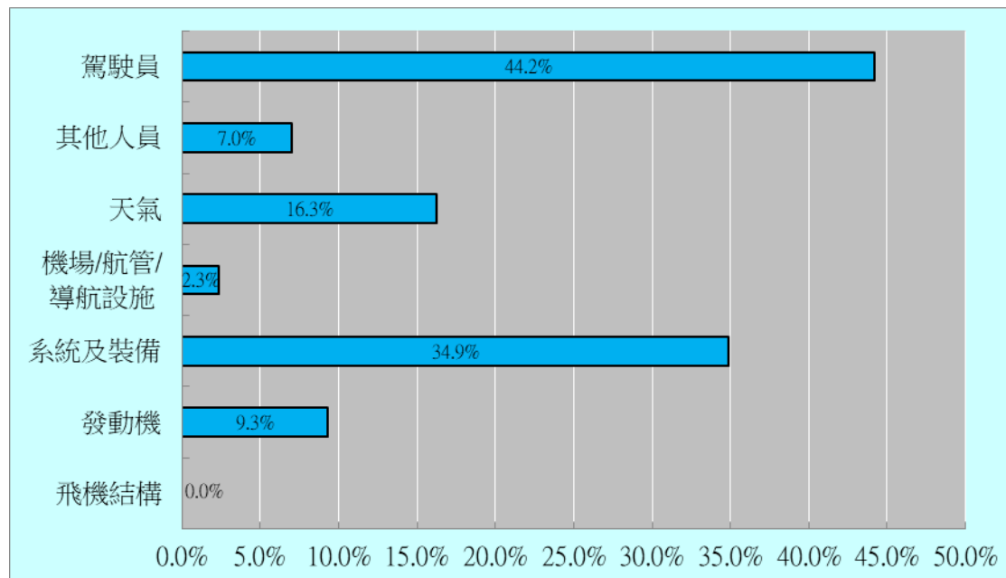
圖15： 2007-2016年國籍民用航空運輸業飛航事故發生原因分類統計
