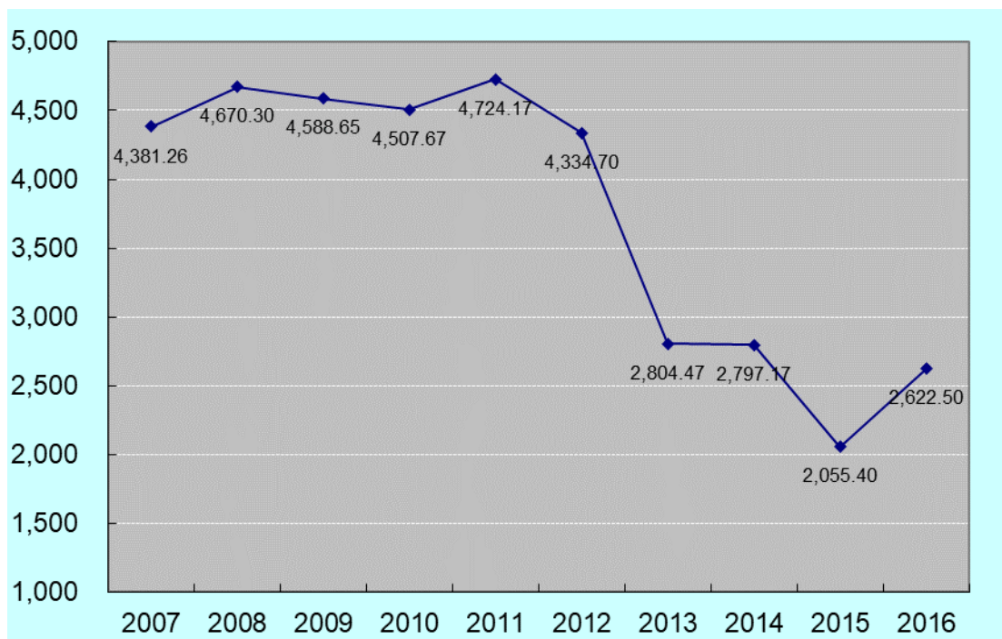
圖6：2007-2016 年間我國普通航空業飛行小時變化圖
