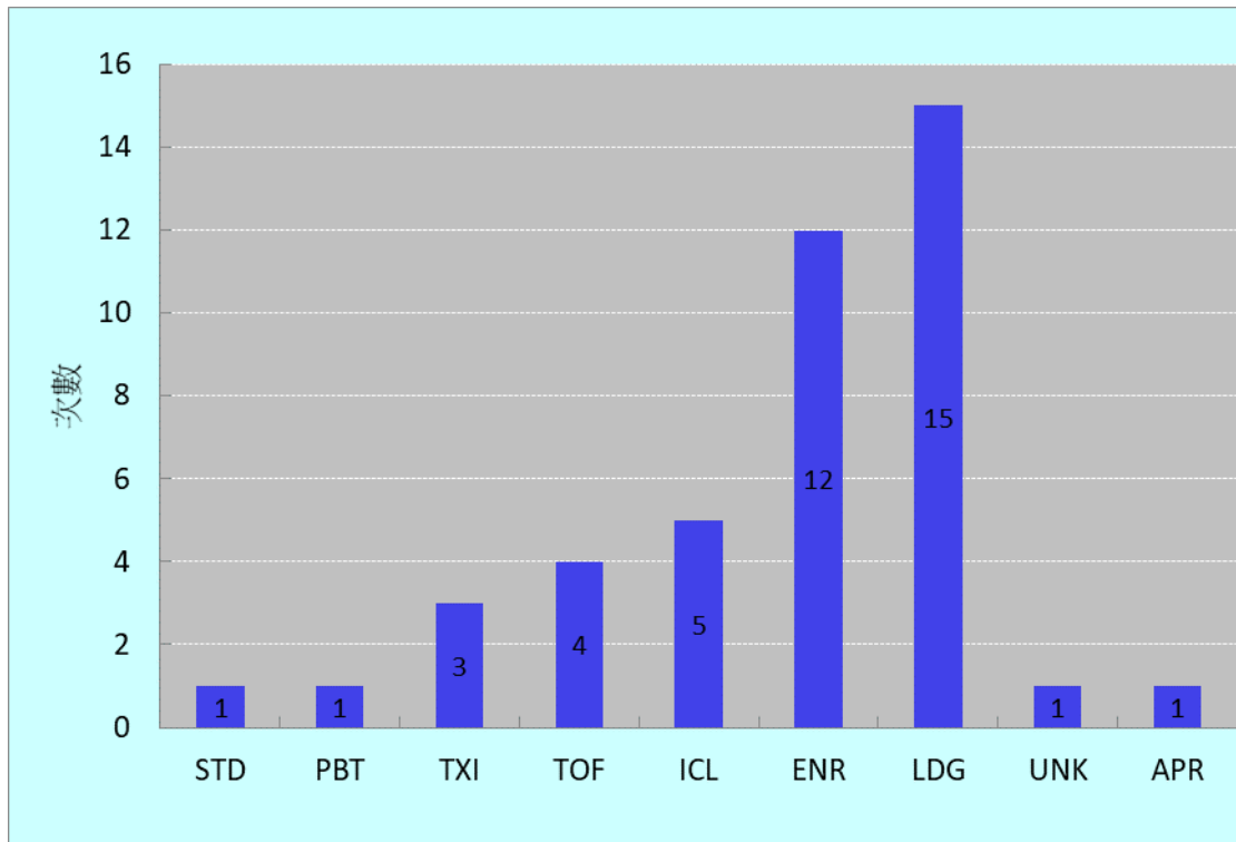
圖13： 2007-2016 年國籍民用航空運輸業飛航事故發生飛航階段次數
