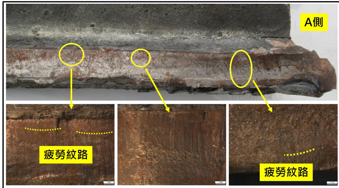
圖 1.14-5 失效件斷裂面 A 側顯微檢視
