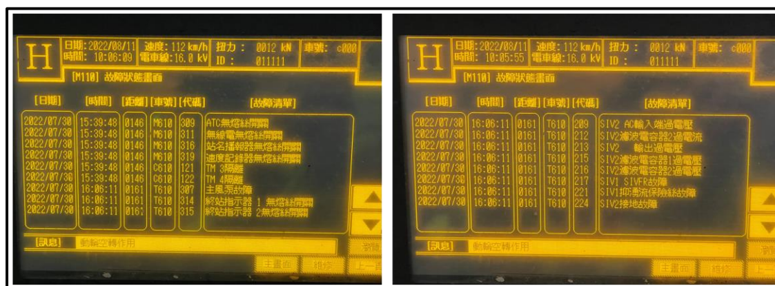
圖 1.10-3 事故列車故障歷史紀錄
