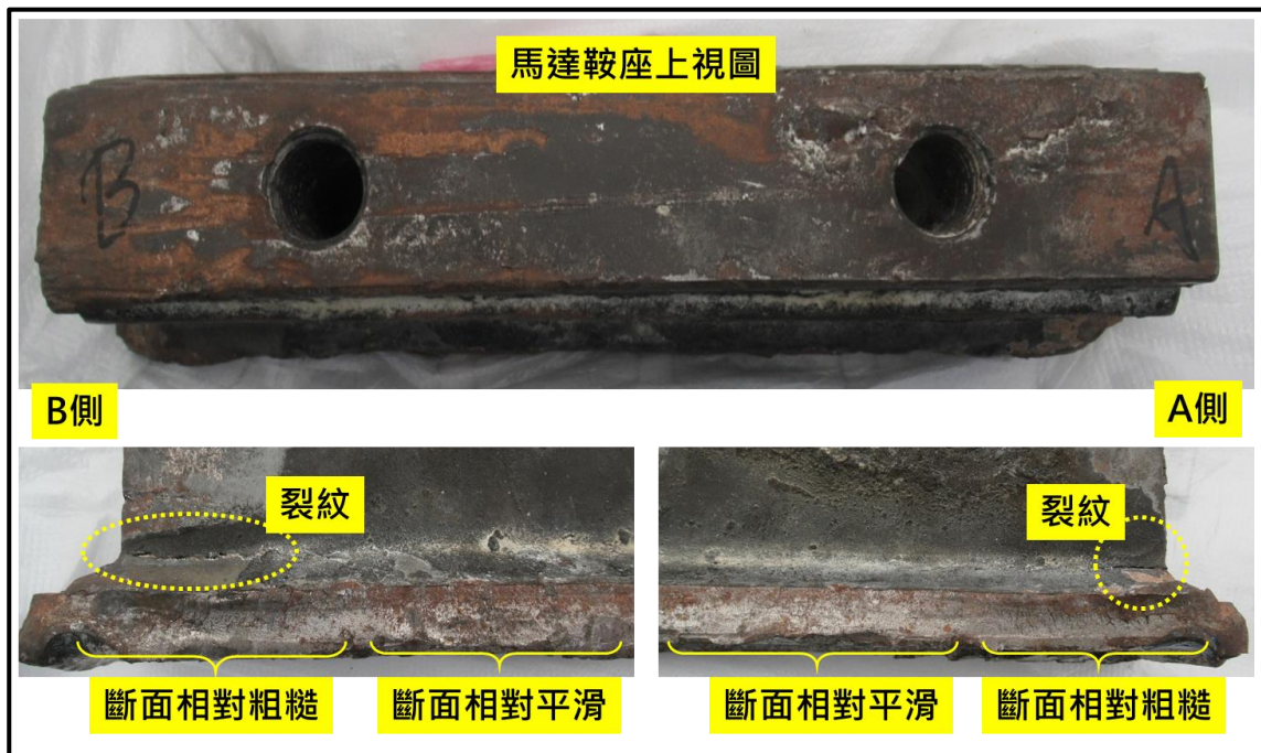
圖 1.14-4 失效件斷裂面 A、B 側目視檢查
