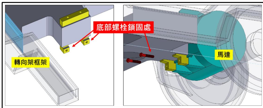
圖 1.5-7 EMU600 型電聯車馬達底部螺栓鎖固處
