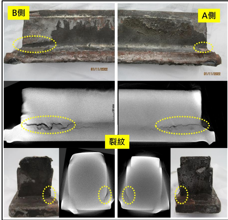
圖 1.14-9 失效件電腦斷層影像
