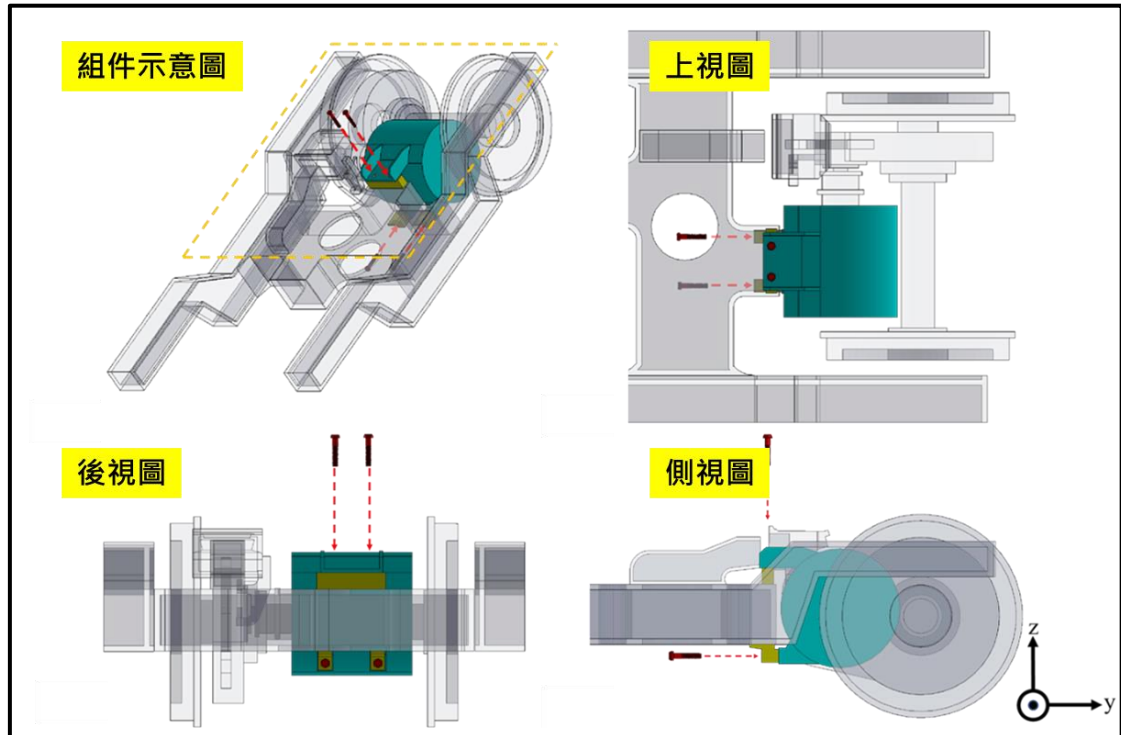
圖 1.14-2 EMC610 號轉向架實體模型
