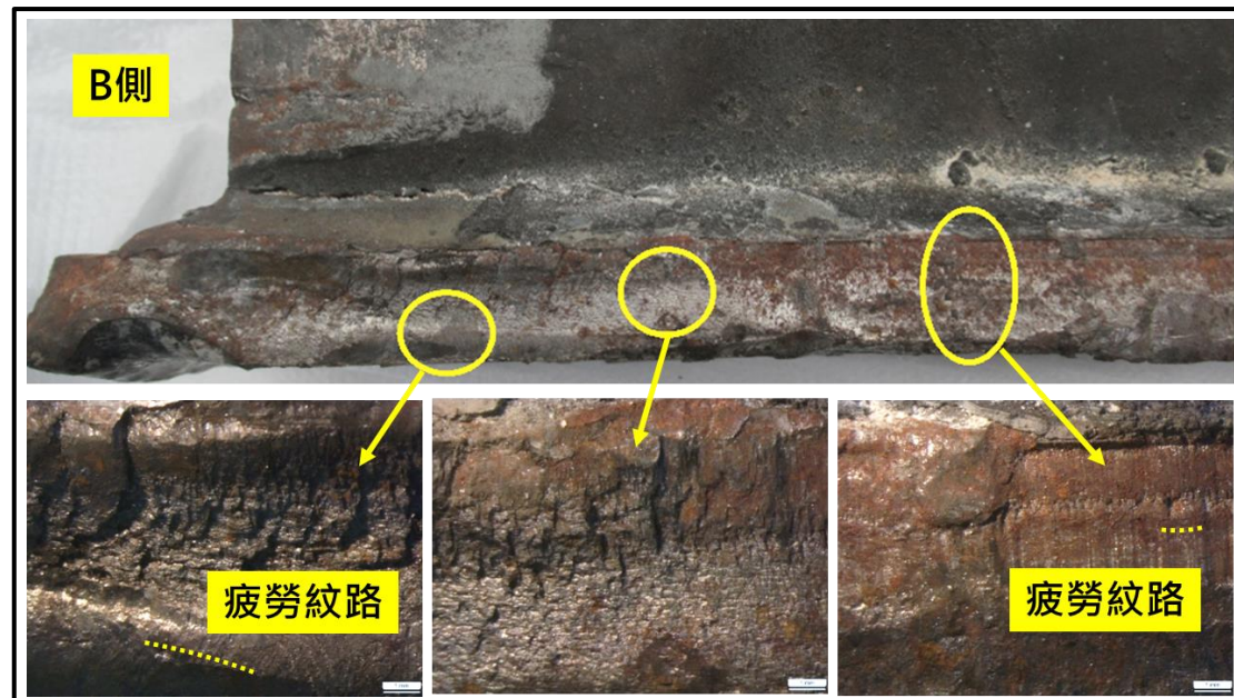
圖 1.14-6 失效件斷裂面 B 側顯微檢視
