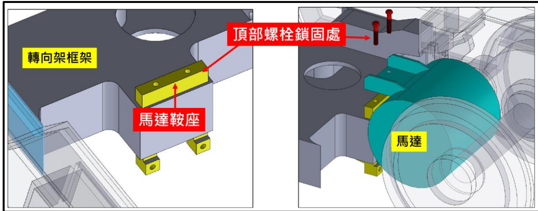
圖 1.5-6 EMU600 型電聯車馬達頂部螺栓鎖固處
