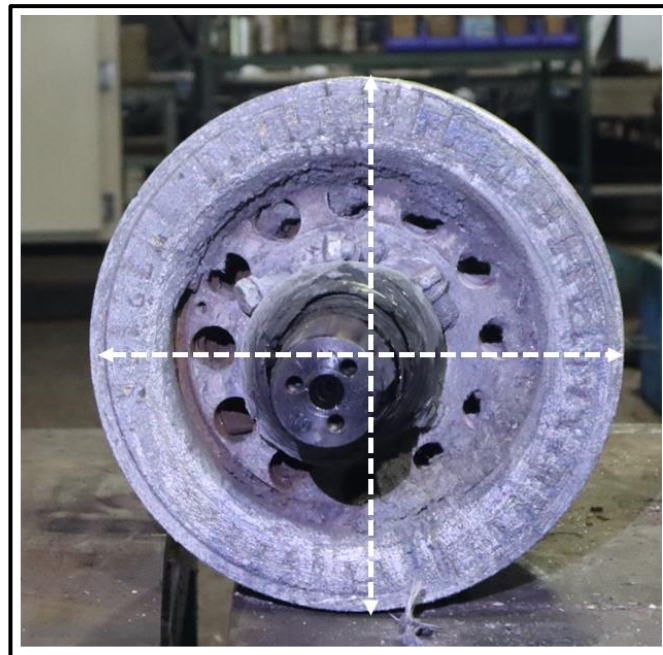
圖 1.11-11 事故馬達轉子與齒輪箱連結軸端
