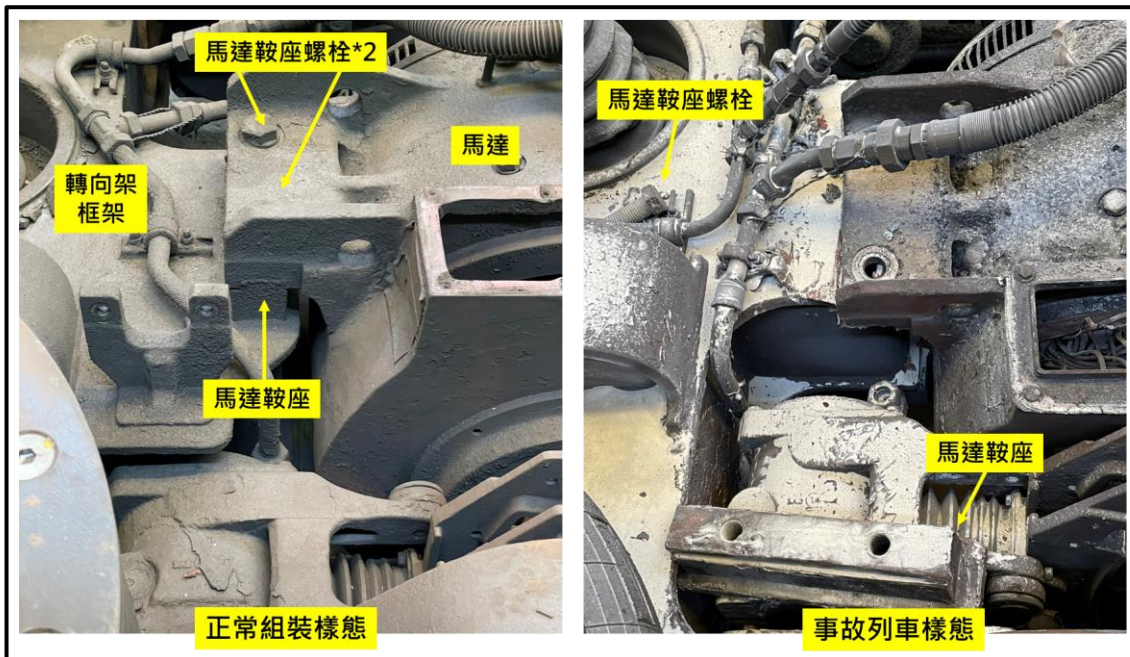
圖 1.11-3 馬達與轉向架組裝處對照
