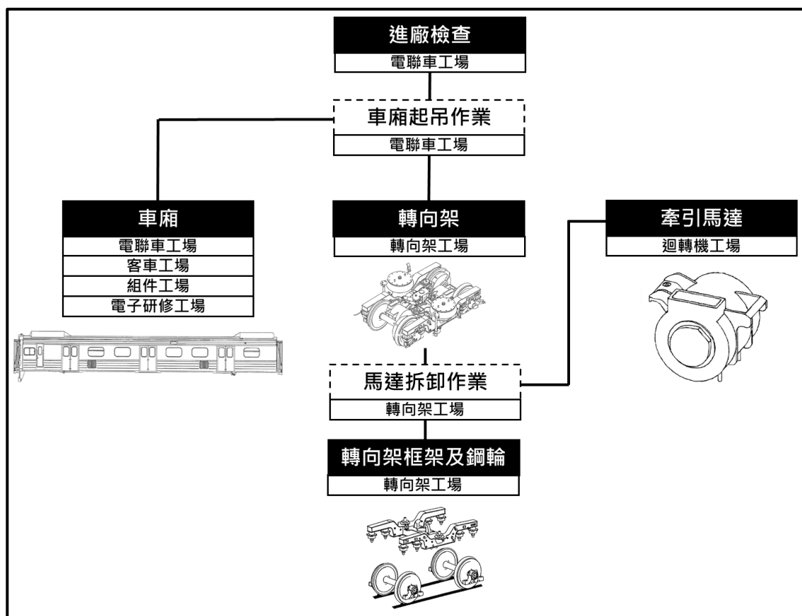
圖 1.15-1 EMU600 型電聯車三、四級檢修馬達拆卸流程
