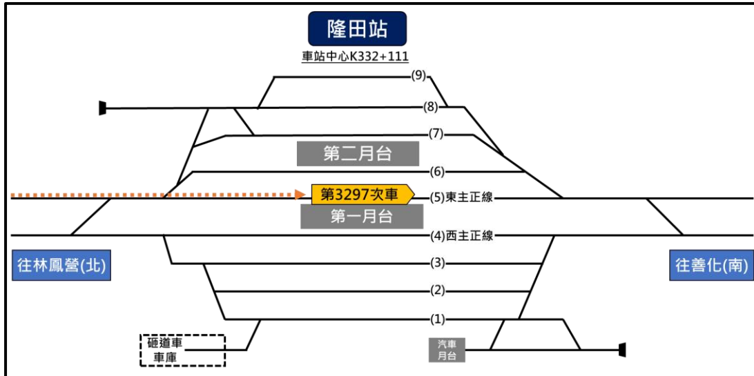
圖 1.1-2 隆田站路線及月台配置圖
