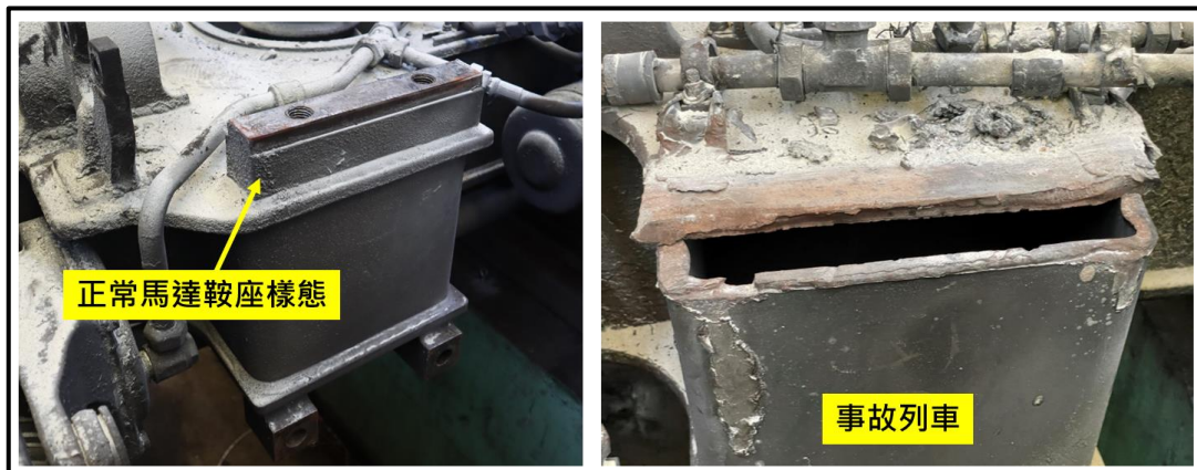
圖 1.11-6 馬達鞍座對照圖
