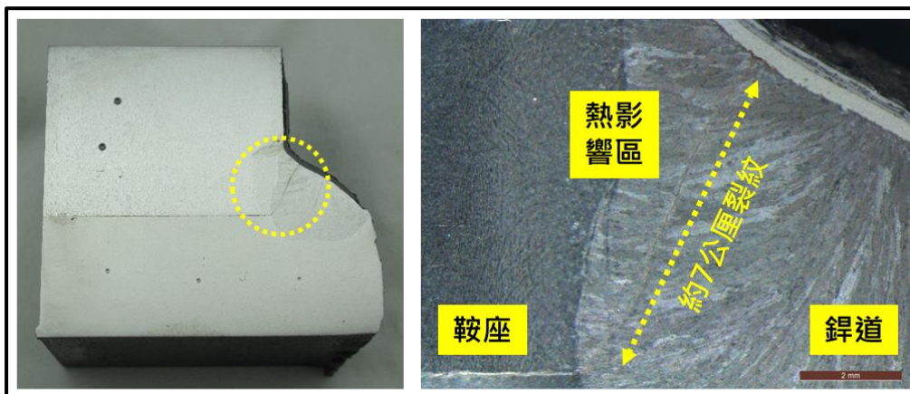
圖 1.14-13 斷裂側金相分析
