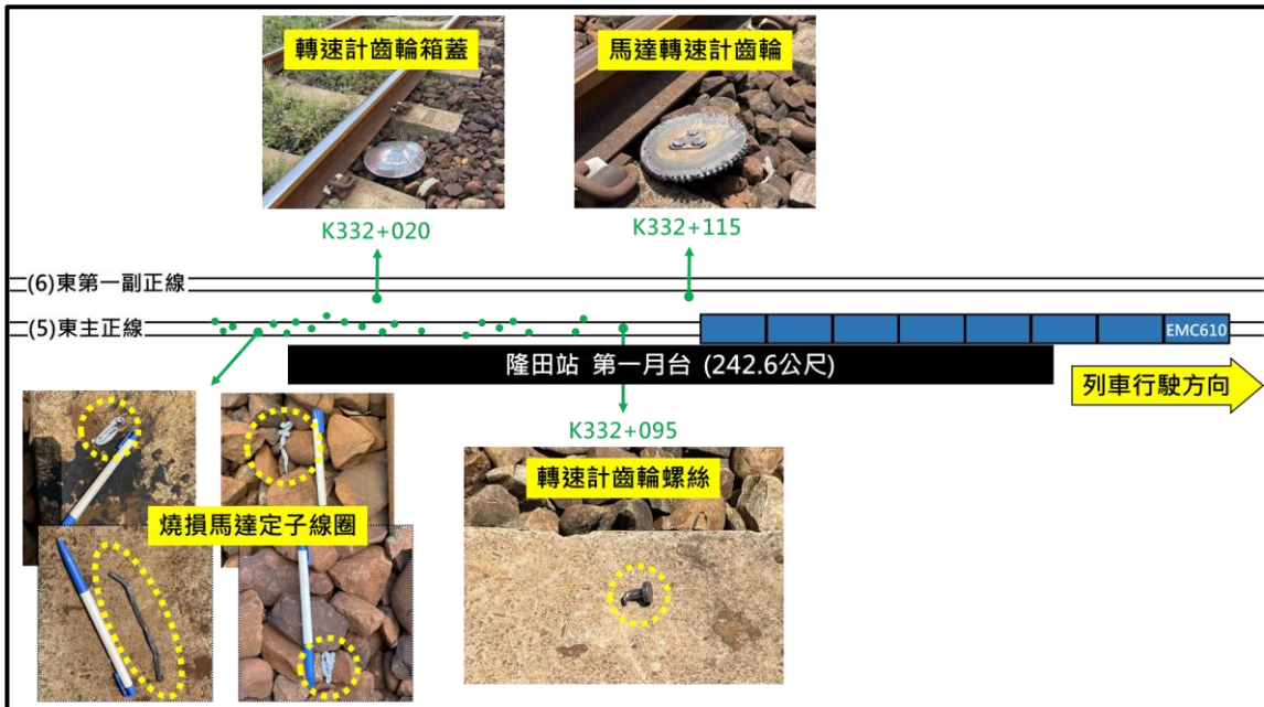
圖 1.3-4 事故列車停放位置與零件分布相對位置
