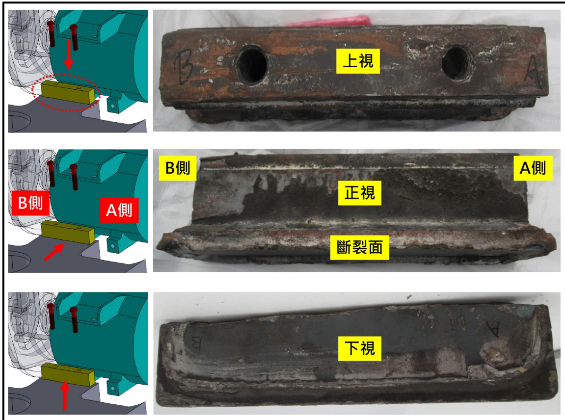
圖 1.14-3 失效件上視、正視及下視圖
