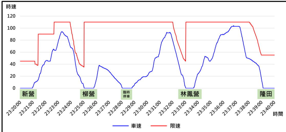
圖 1.10-1 事故列車 ATP RU 資料
