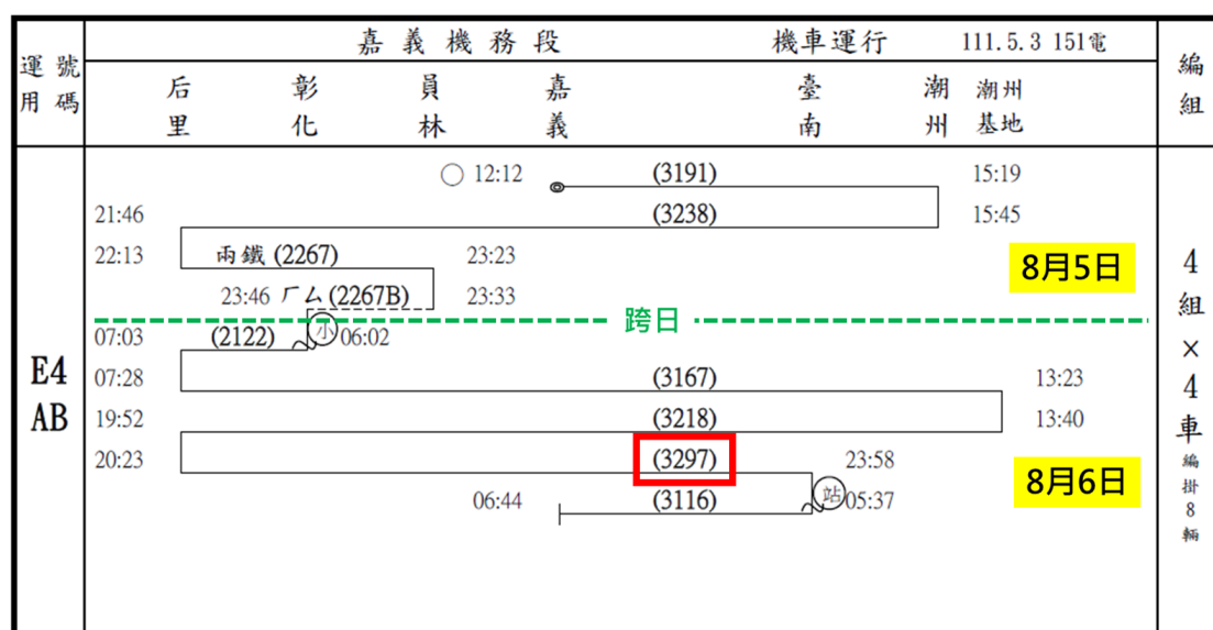
圖 1.5-2 EMU610 號編組運用情形
