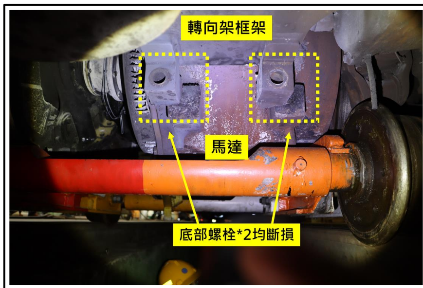
圖 1.11-5 馬達與轉向架組裝處對照
