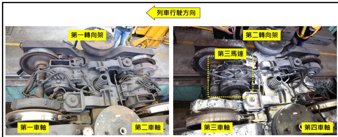
圖 1.11-1 第一轉向架與第二轉向架比較
