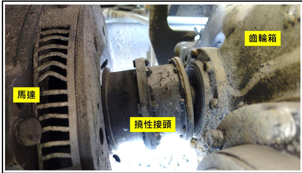
圖 1.3-3 第二轉向架之第三馬達撓性接頭位移
