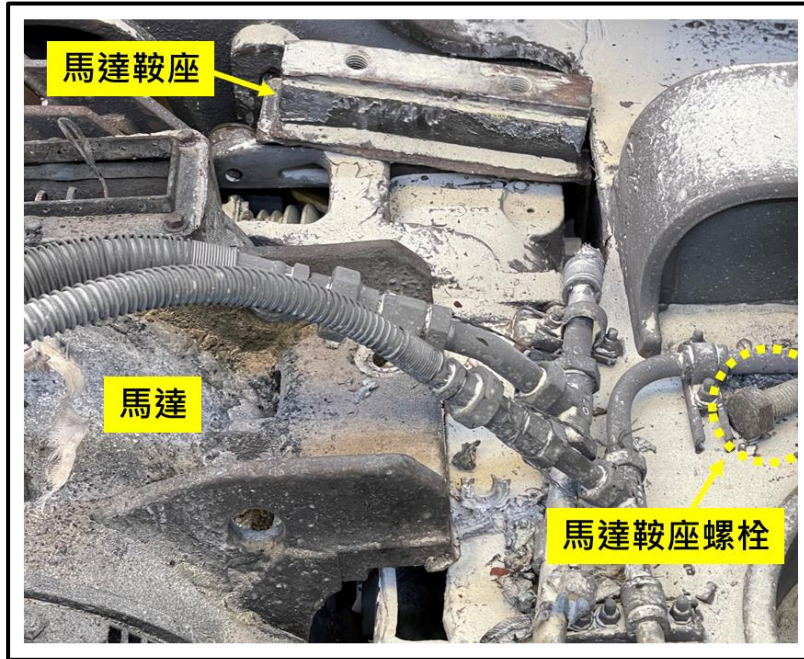
圖 1.11-2 第三馬達鞍座斷裂情形
