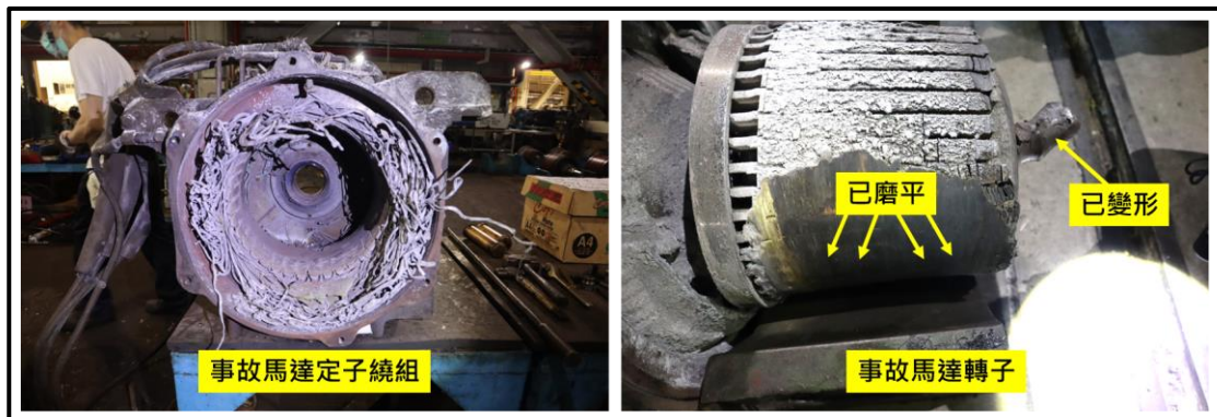
圖 1.11-9 事故馬達定子及轉子
