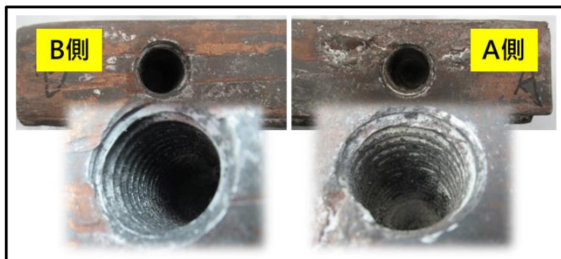
圖 1.14-8 失效件上螺孔檢視
